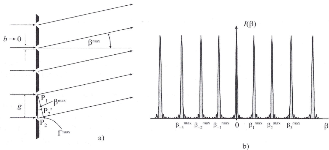
Abb. 3: Fraunhofer-Beugung am idealen Gitter a) Zur Entstehung der Beugungsmaxima b) Intensitätsverteilung des idealen Amplitudengitters
