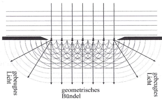
Abb. 1: Huygens-Fresnel'sches Prinzip
