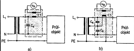
Einkopplung von a) Gegentaktstörungen b) Gleichtaktstörungen
