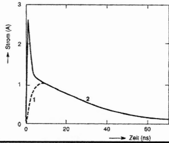
Doppelt exponentieller Impulsverlauf
